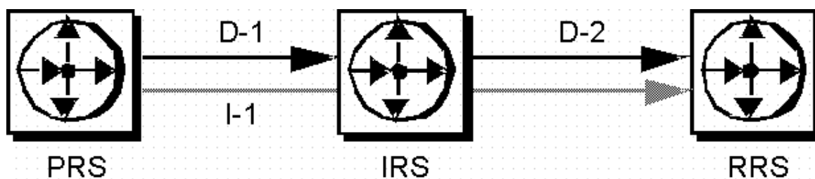
图 4: 直接路由和间接路由示例
